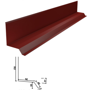
20. Stänkleck
