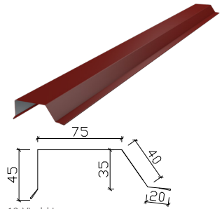
12. Vindskiva
