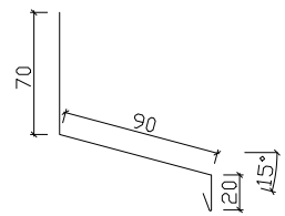
5-6. Överbleck 90
