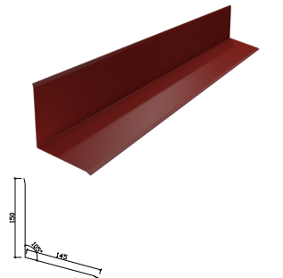
17-19. Stänkleck
