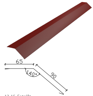
13-15. Fotplåt
