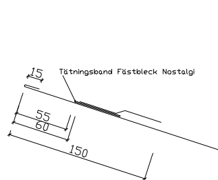
21. Ränn dal Nostalgi detalj
