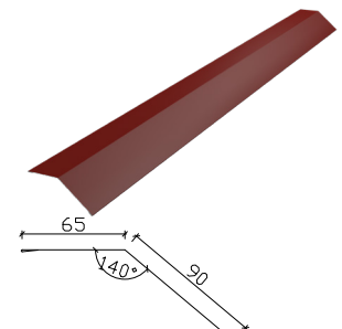
13-15. Fotplåt
