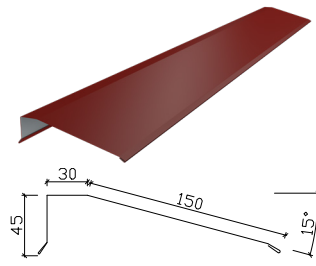
6-8. Pulpetnock
