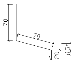
3-4. Överbleck 70
