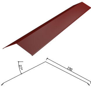
1-3. Nockhuv 155, 190
