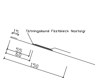
21. Rännål Nostalgi detalj
