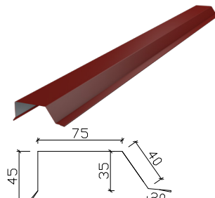
12. Vindskiva
