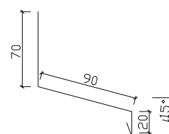
5-6. Överbleck 90
