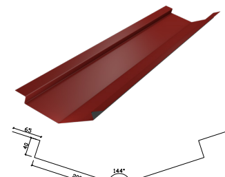
22. Rännål
