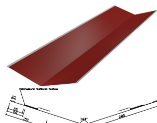
21. Rännål Nostalgi
