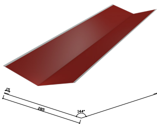
21. Rännål
