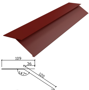
16. Fotplåt
