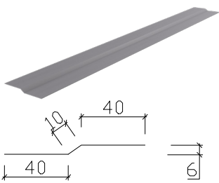
23. Fästbleck rännål Nostalgi
