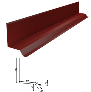
20. Stänkebleck
