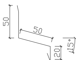
1-2. Överbleck 50
